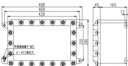
最大取付端子数 (20A 端子台の場合) 32P×2列
