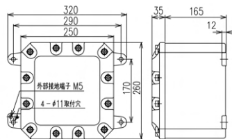
最大取付端子数 (20A 端子台の場合) 12P×2列
