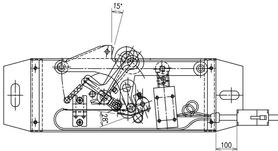
取付外形寸法図
