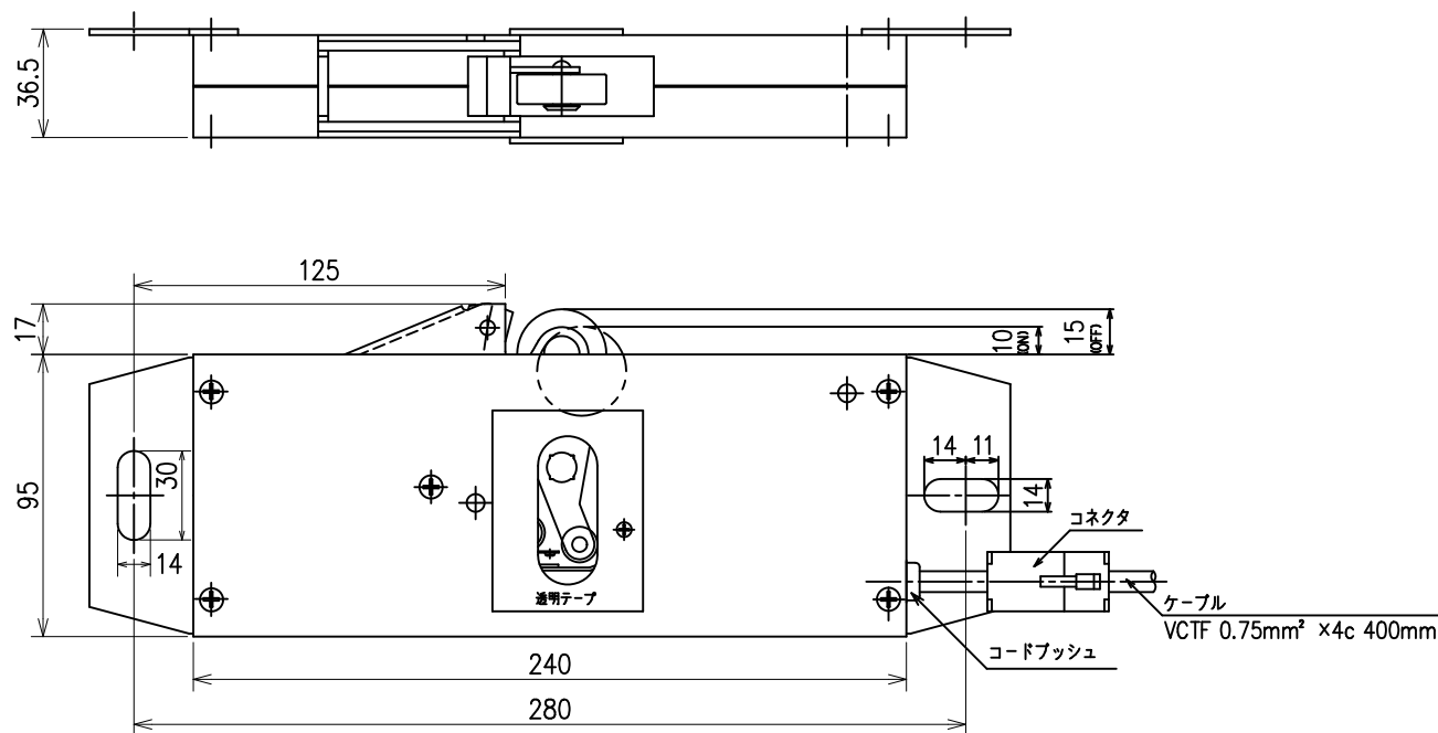
取付外形寸法図
