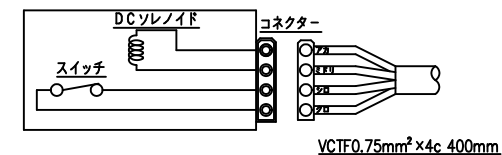
配線図
