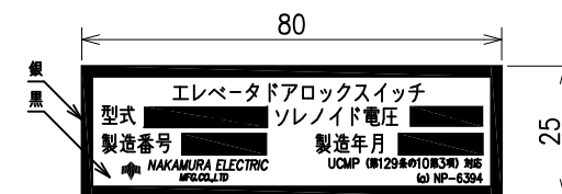
定格銘板詳細図
