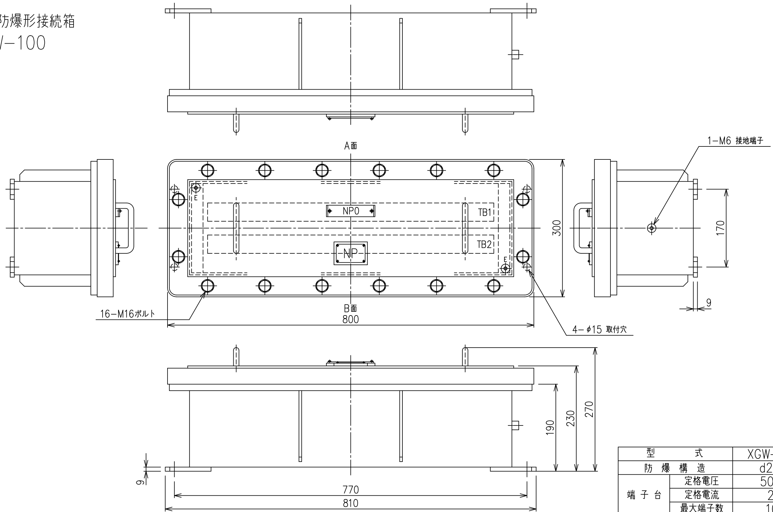
外部導線引込み器具最大取付個数 (一つの面)
