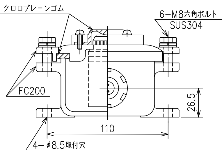
貫通金物 F-8801
