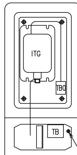
盤内器具配置図
